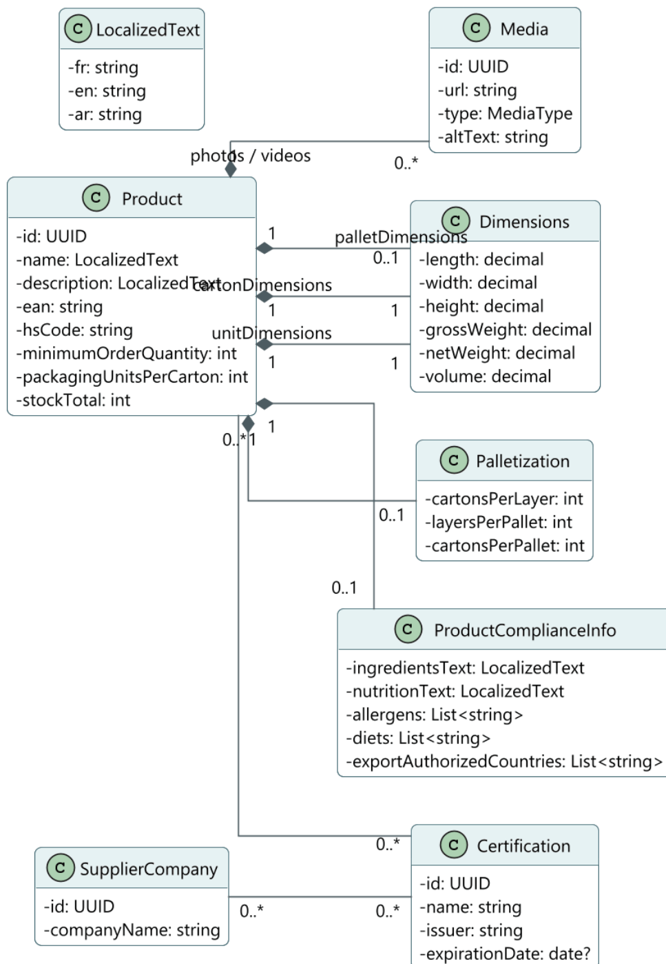
FIGURE 3 – Diagramme de classes - détail du catalogue produit
