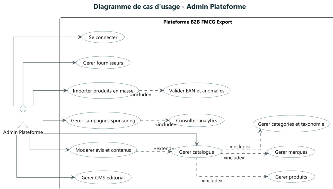
FIGURE 8 – Cas d’usage - administrateur
