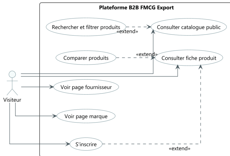
FIGURE 4 – Cas d'usage - visiteur
