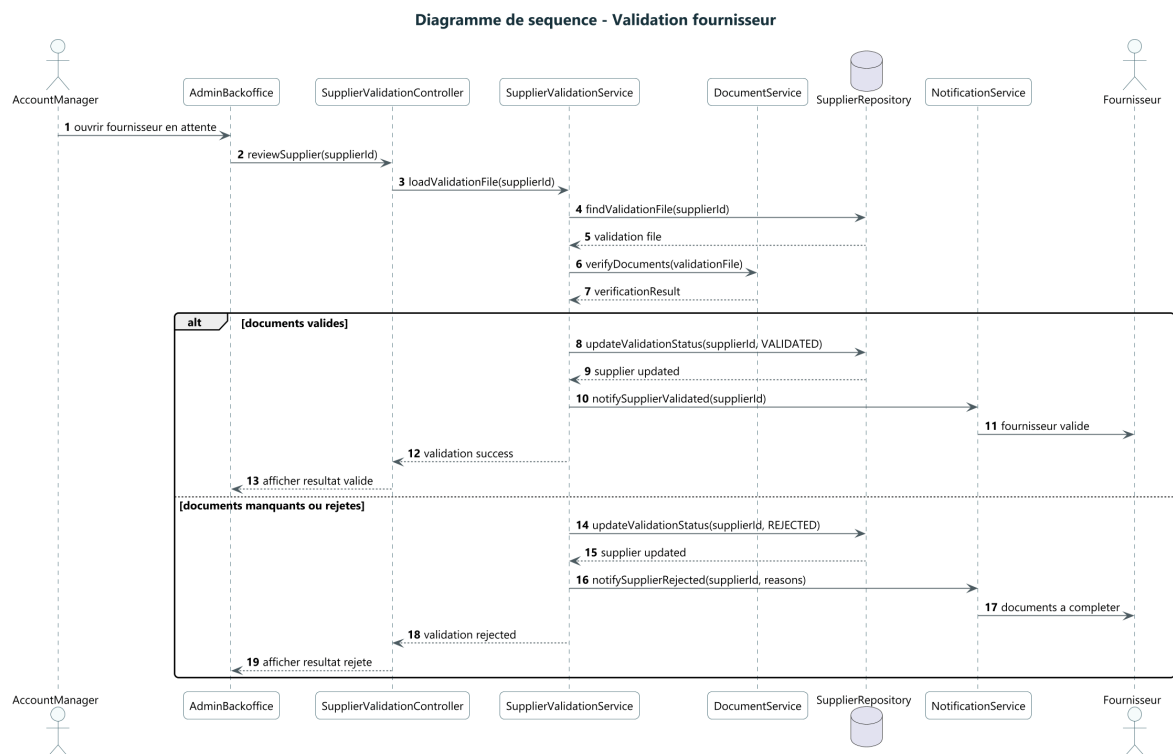
FIGURE 12 – Séquence - validation d'un fournisseur
