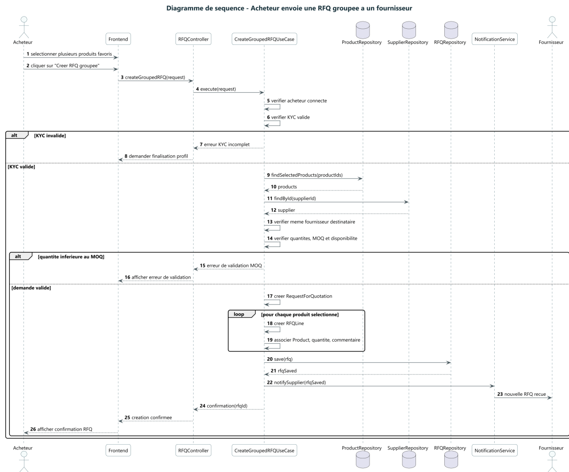
FIGURE 10 – Séquence - création d'une RFQ groupée
