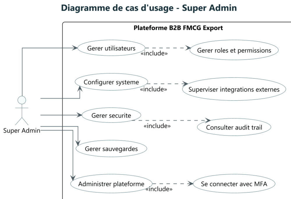
FIGURE 9 – Cas d’usage - super administrateur
