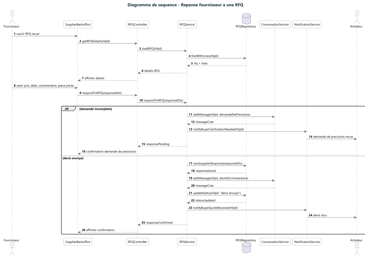
FIGURE 11 – Séquence - réponse du fournisseur à une RFQ
