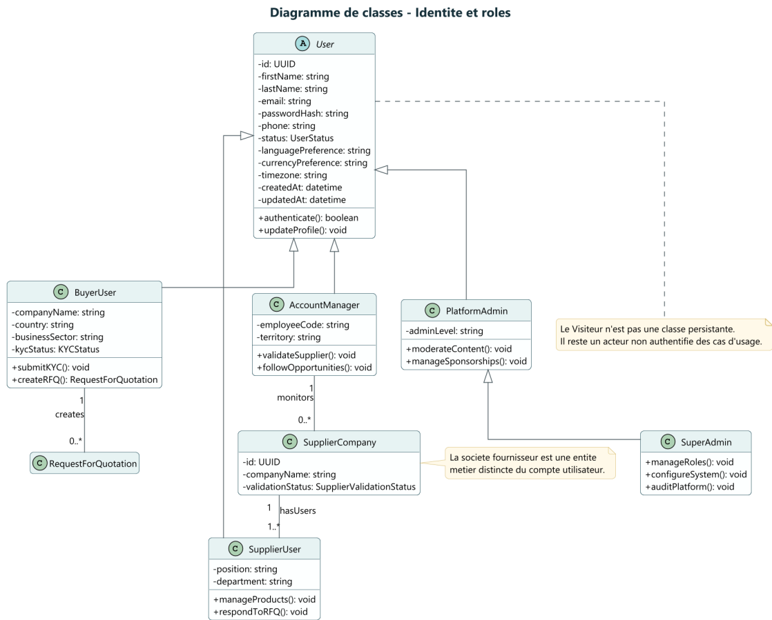
FIGURE 2 – Diagramme de classes - rôles et identités
