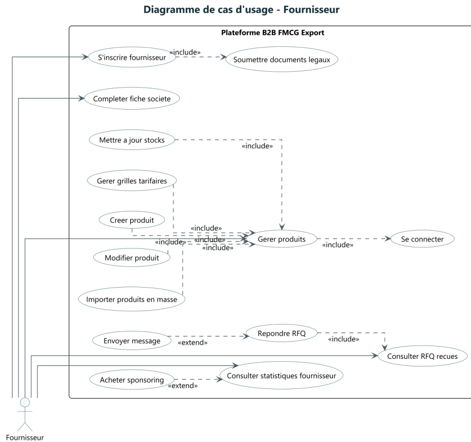
FIGURE 6 – Cas d'usage - fournisseur
