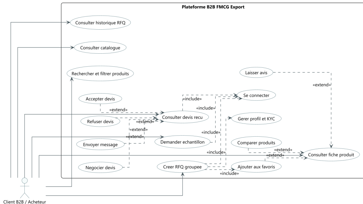
FIGURE 5 – Cas d'usage - client / acheteur
