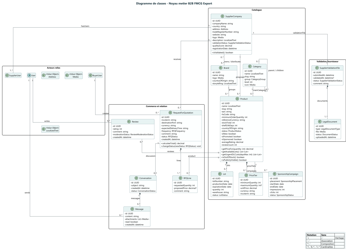
FIGURE 1 – Diagramme de classes - domaine métier principal
