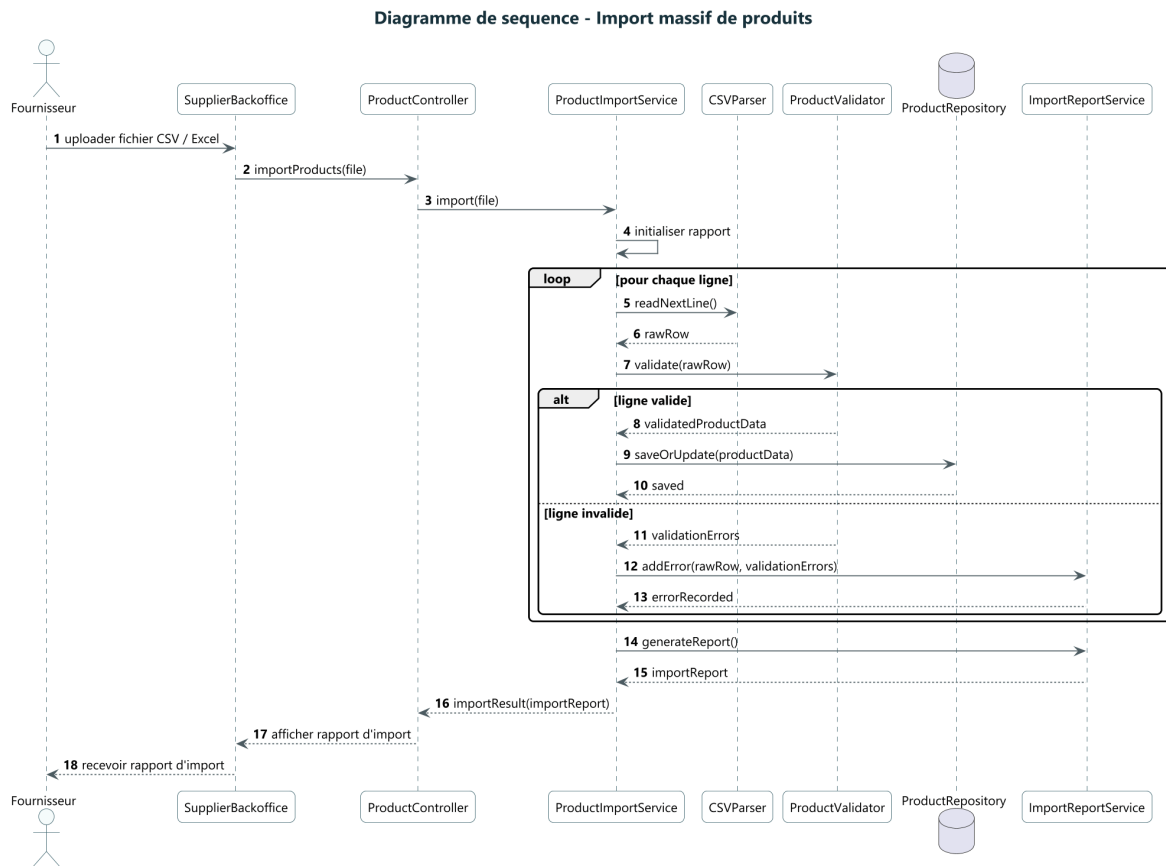
FIGURE 13 – Séquence - import massif de produits
